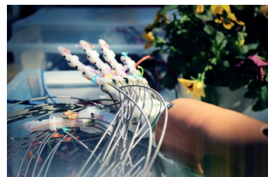
進化系ロボットアーム「筋電義手」
