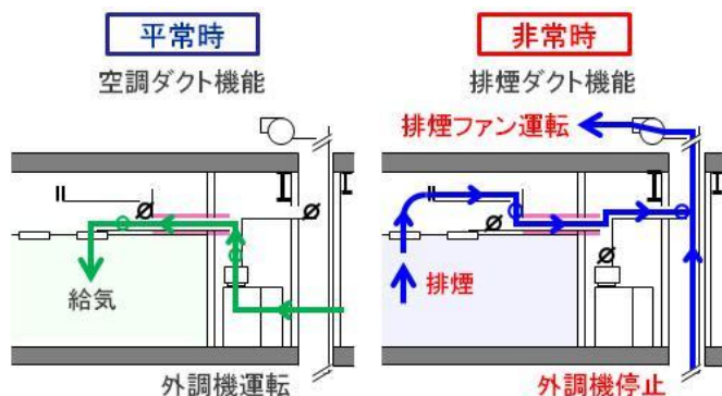
空調ダクト兼用加圧防煙設備。平常時と火災等の緊急時で空調ダクトと排煙ダクトを切り換えられるようにした。
